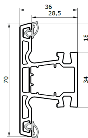
POSTE DZ 36
